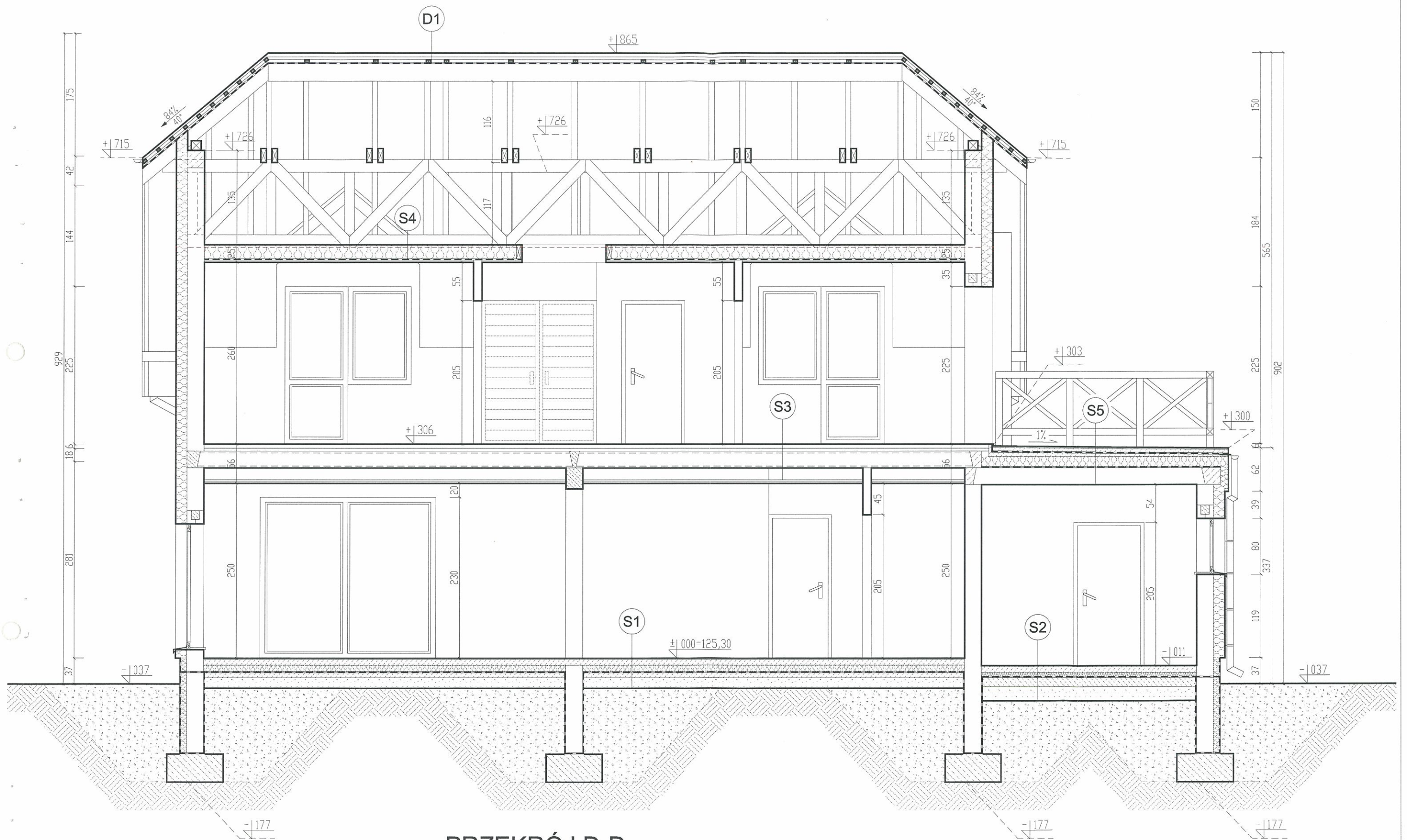
PRZEKRÓJ D-D
